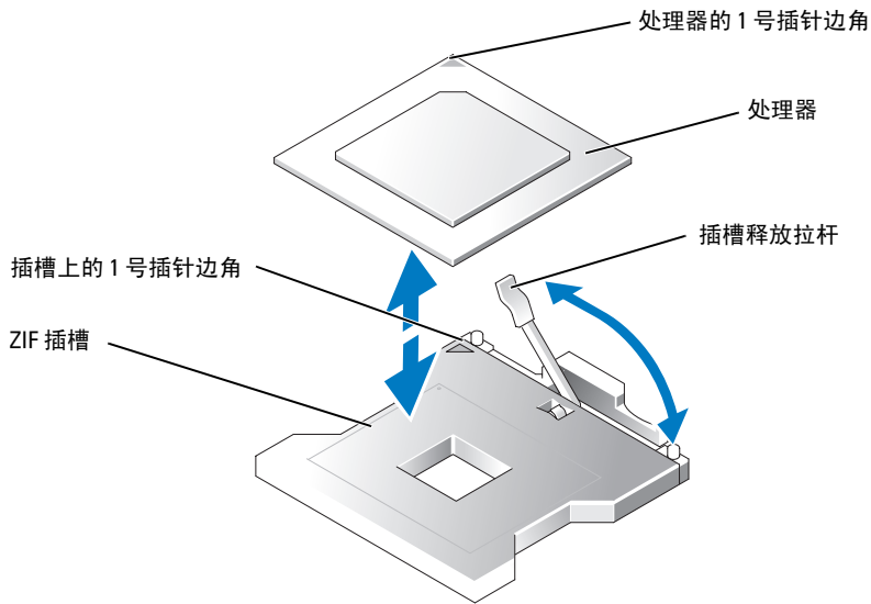
图 1-2. 装卸处理器
