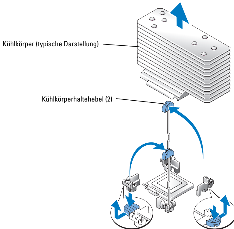
Abbildung 1-1. Kühlkörper entfernen und installieren
